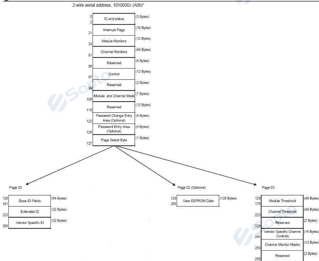
Figure4. QSFP Memory Map
